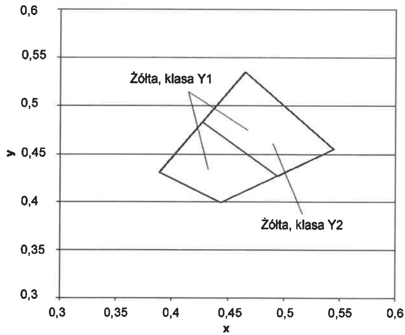
Rys.2. Współrzędne chromatycności x,y dla barwy żółtej oznakowania
