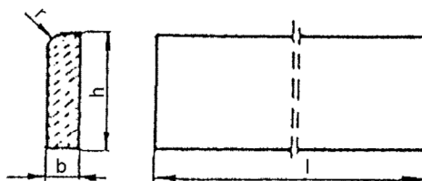
Ryśunek 1. Kształt betonowego obrzeża chodnikowego
